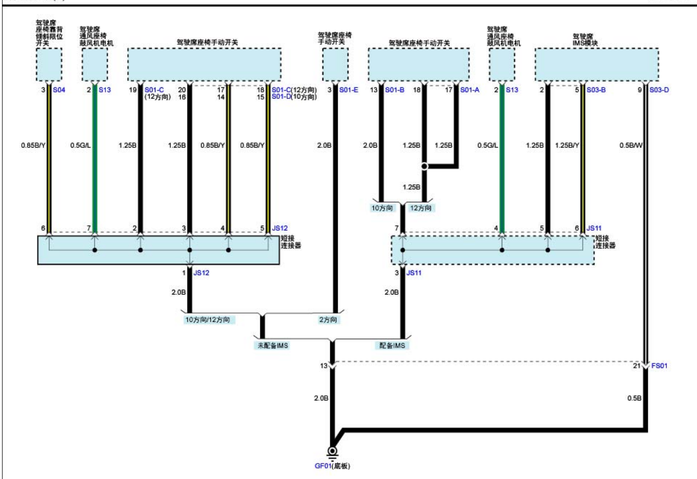
搭铁分布(9)
